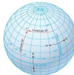
Figura 3. Meridianët dhe paralelet
