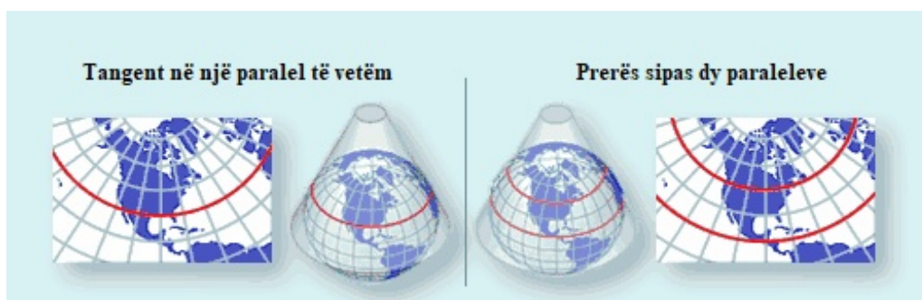
Figura 11. Projeksioni Konik Konform i Lambertit
