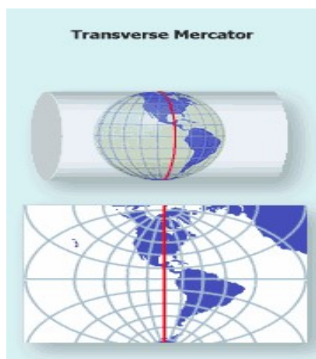
Figura 8. Projeksioni Tërthor i Merkatorit
