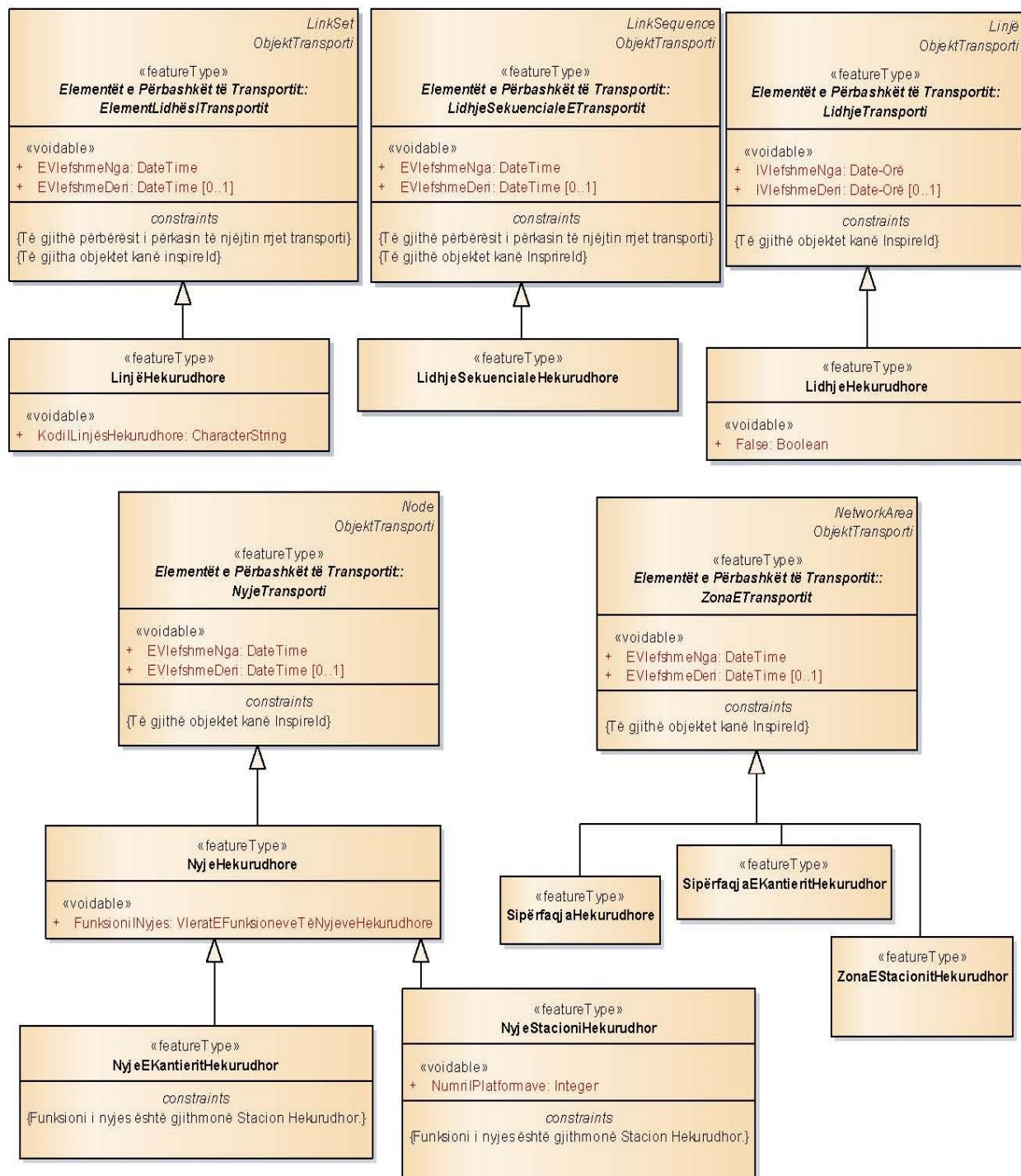
Figure 26: Rrjeti i Transportit Hekurudhor : Llojet e objekteve gjeohapësinore - Lidhjet, Nyjet dhe Zonat
