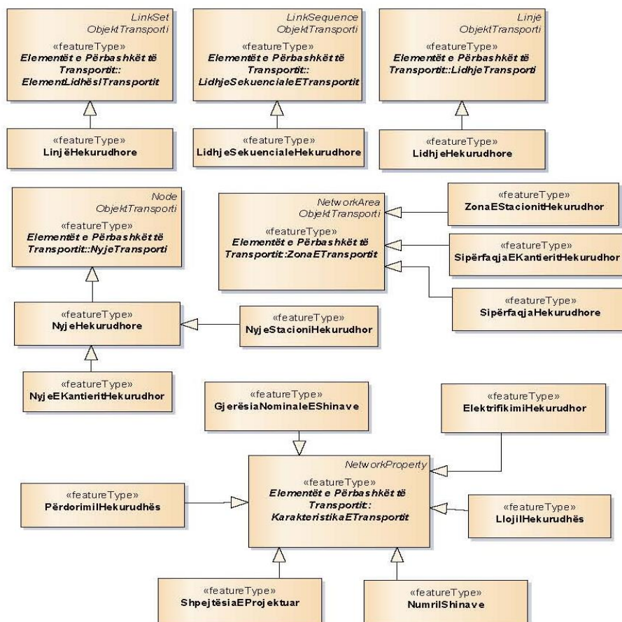
Figure 28: Rrjeti i Transportit Hekurudhor : Pamja e përgjithshme
